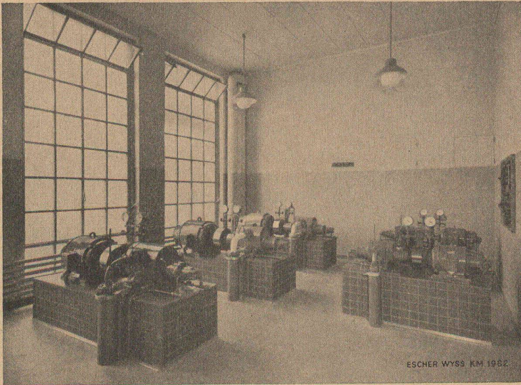
5 compresseurs «ROTASCO» pour la réfrigération des entrepôts frigorifiques
