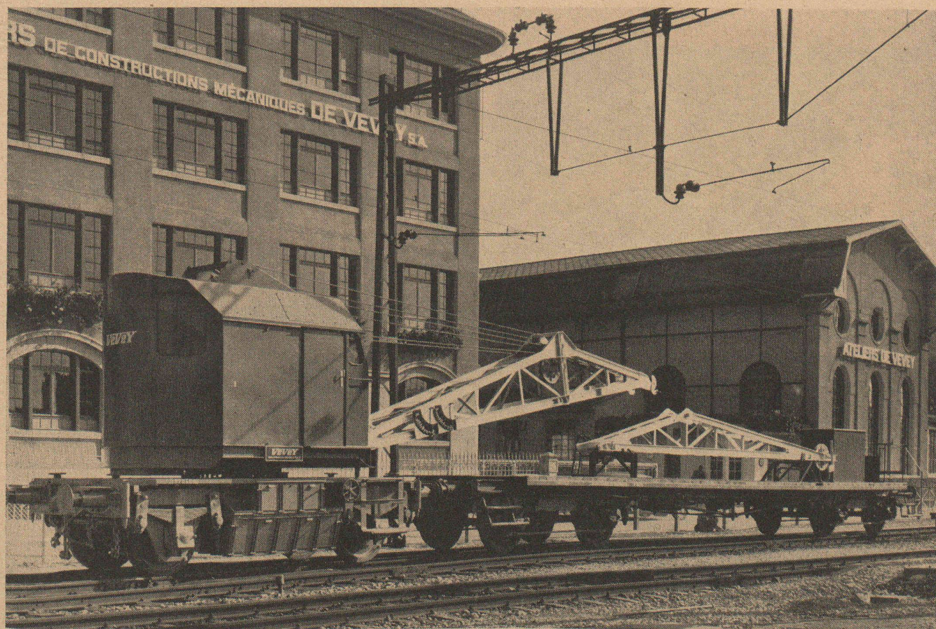
Wagon-grue pour entretien des installations électriques de voies. — Ateliers de Constructions mécaniques de Vevey S. A.
