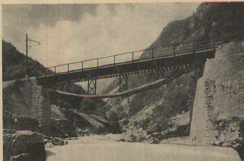
PONT-RAIL DE KIPFEN (Viège-Zermatt) portée 31 m. environ largeur 4 m.
