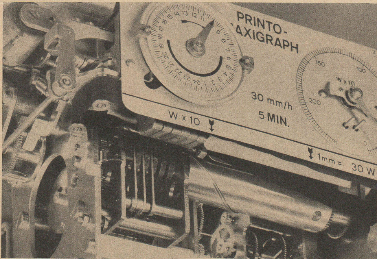
Mécanisme d'un enregistreur-imprimeur « Printo-Maxigraph » de LANDIS & GYR S. A., Zoug.
