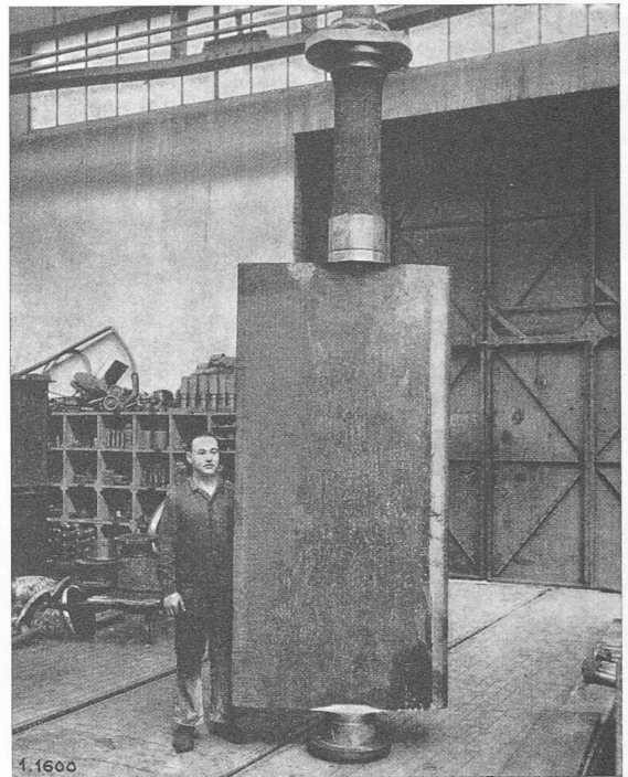
Fig. 24. — Aube directrice.
