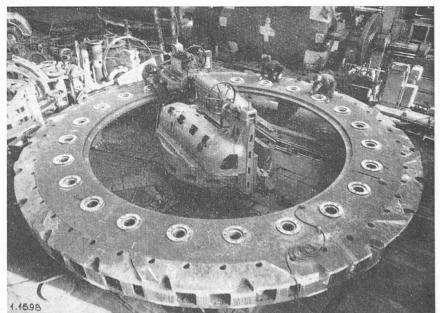
Fig. 17. — Usinage du fond annulaire et couronne inférieure de l'anneau d'entretoises, dans les ateliers d'Alsthom, à Belfort.
