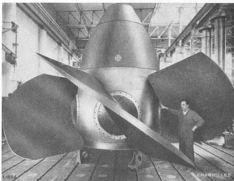
Fig. 20. — Roue motrice entièrement montée, en ateliers.
