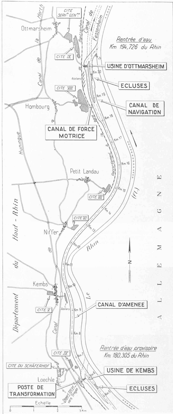
Fig. 3. — Tracé du canal entre les centrales de Kembs et d'Ottmarsheim.
