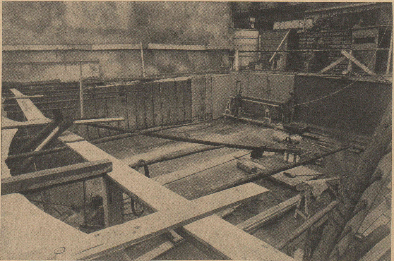
Isolation et étanchéité des fondations de l'immeuble de la COMPAGNIE D'ASSURANCE NATIONALE SUISSE à GENÈVE
