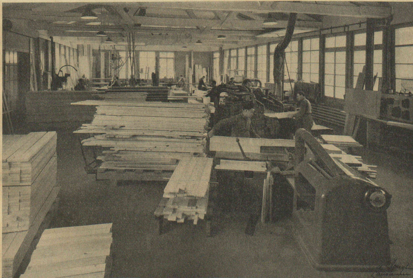
Vue de l'atelier d'usinage de la Fabrique Coopérative de Menuiserie de Lausanne.
