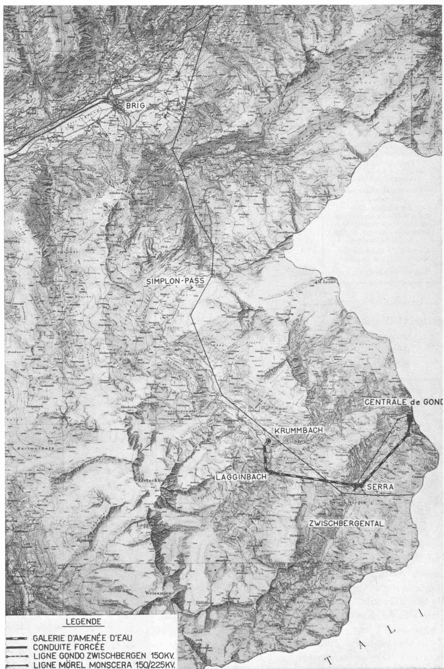
Fig. 1. — Energie électrique du Simplon. — Plan de situation. Echelle 1 : 150 000.
