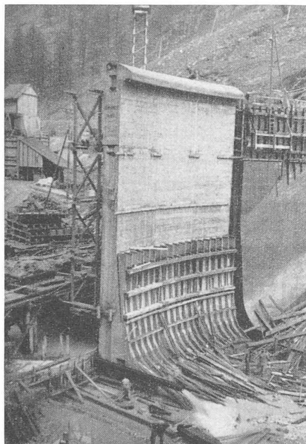
Fig. 3. — Barrage de Serra. Vue côté aval.
