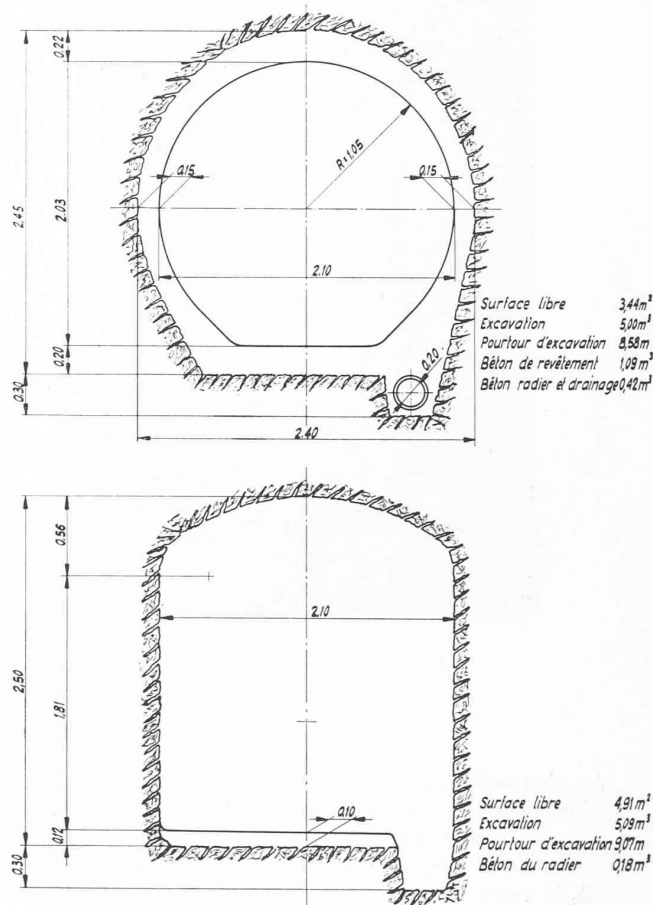
Fig. 2. — Coupes transversales de la galerie sous pression revêtue et de la galerie à veine libre.
