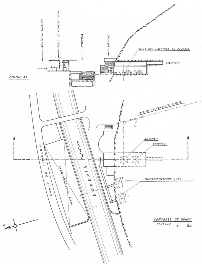
Fig. 6. — Centrale de Gondo. — Plan de situation.
