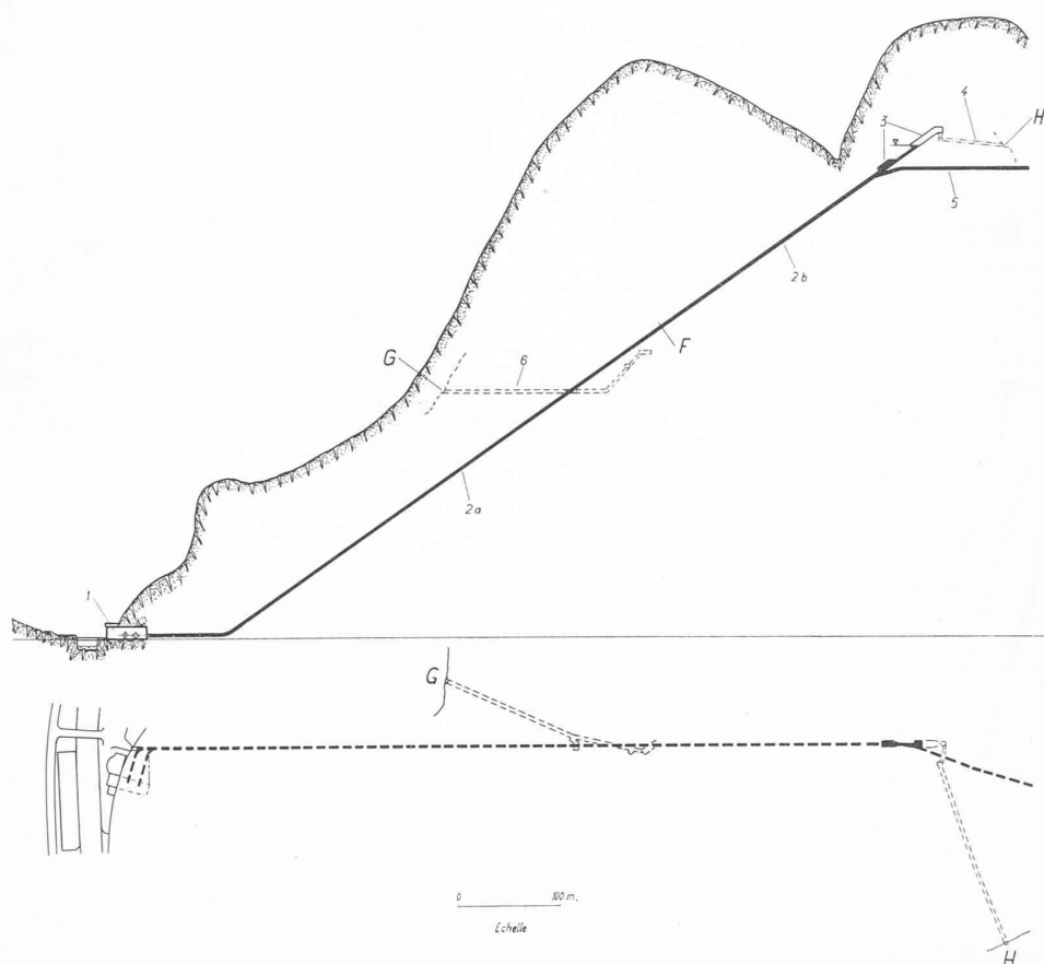
Fig. 5. — Centrale de Gondo. — Chambre d'équilibre et puits incliné.
