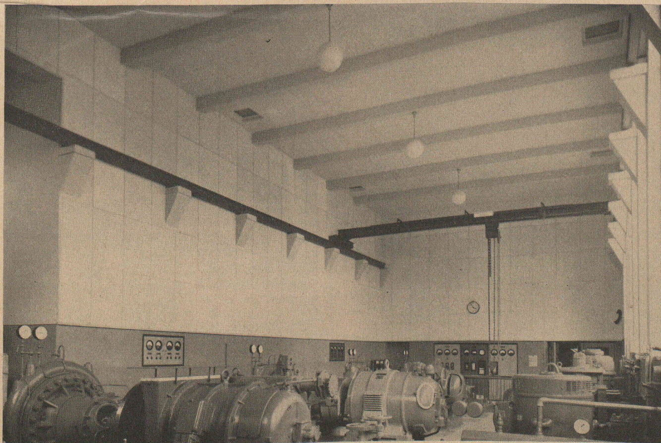
Station de pompage du Service des Eaux de la Ville de Lausanne, à Lutry. Absorption du bruit dans la salle des pompes par revêtement de plaques VETROFLEX.
