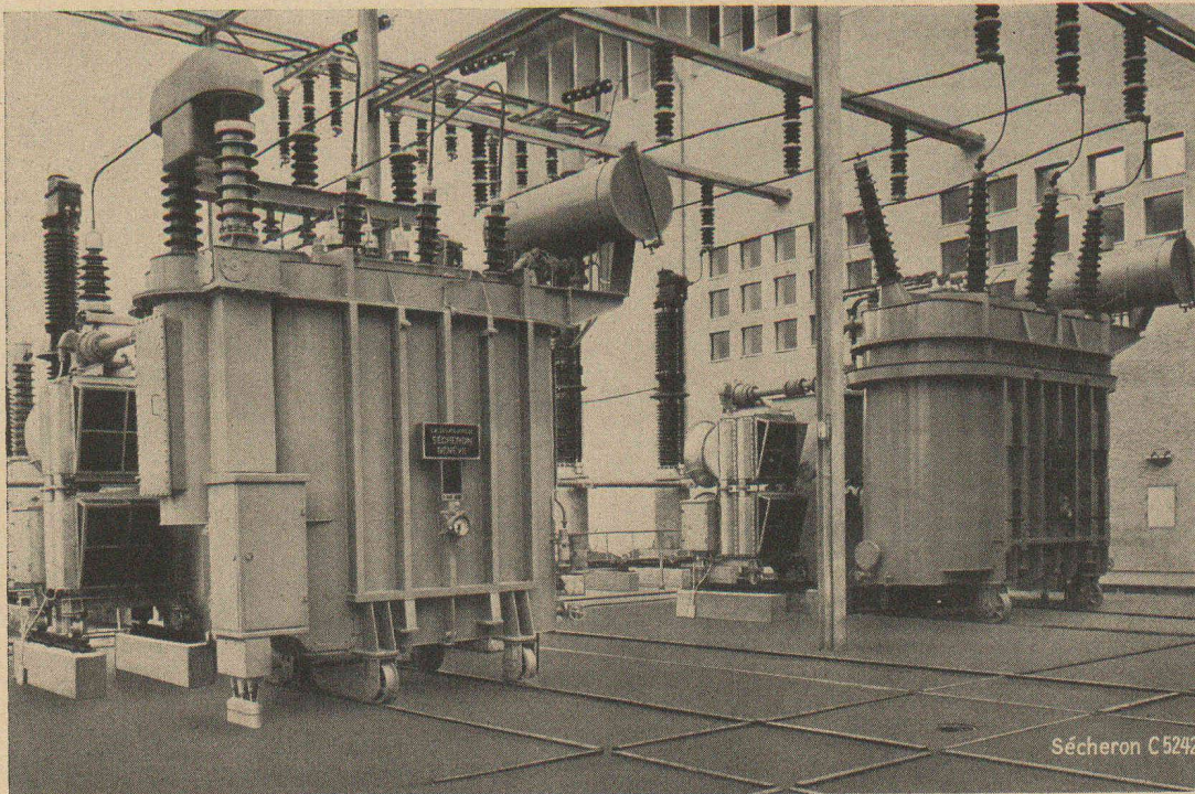
4 transformateurs de 20 000 KVA et 30 000 KVA à la centrale de Wildegg-Brugg (Argovie). Circulation forcée de l'huile dans des radiateurs ventilés. (Nordostschweizerische Kraftwerke A.G. Baden).
