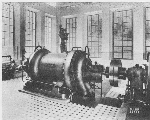
Fig. 4. — Pompe d'accumulation à haute pression de 7500 ch, centrale d'Oberems (Illsee-Tourtemagne).
