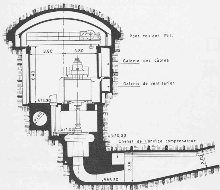
Fig. 7. — Usine. Coupe en travers Echelle 1 : 250.
