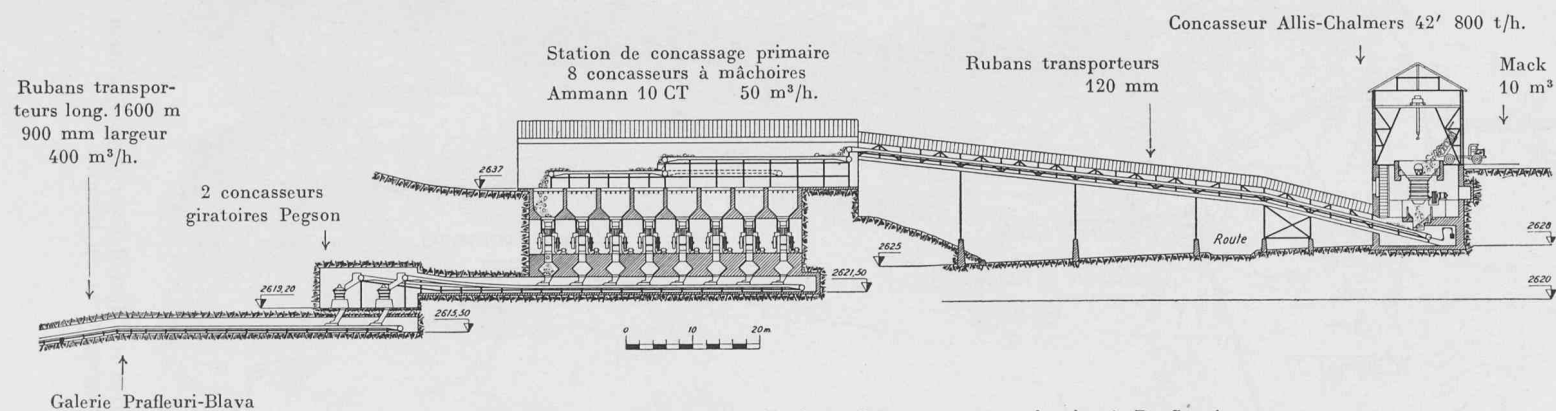
Fig. 4. — Profil en long des installations de concassage primaire à Präfleuri.
