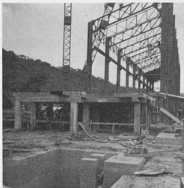
Fig. 6. — Hal du four, côté cuiseur : début montage.
