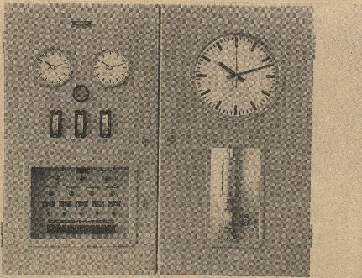
Centrale horaire d'une grande gare de chemins de fer, avec remise à l'heure automatique. Capacité : environ 50 horloges secondaires sur deux circuits.
