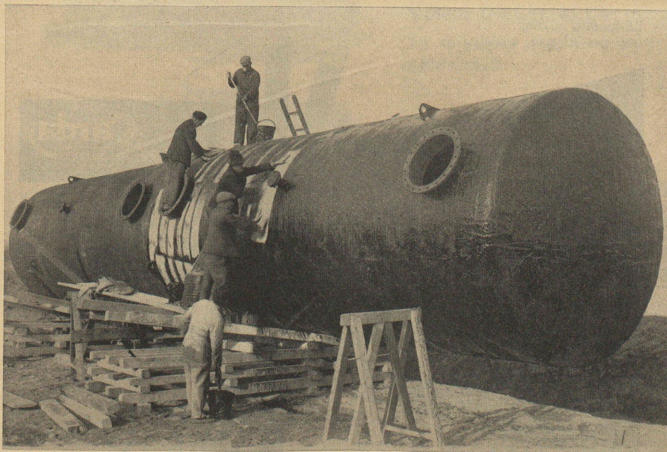
Revêtement anti-corrosif d'une citerne à essence d'une contenance de 150 000 litres, exécuté par la Maison Vve A. HIRSCHY & Cie S. A., 50, Rue de Lausanne, Genève.
