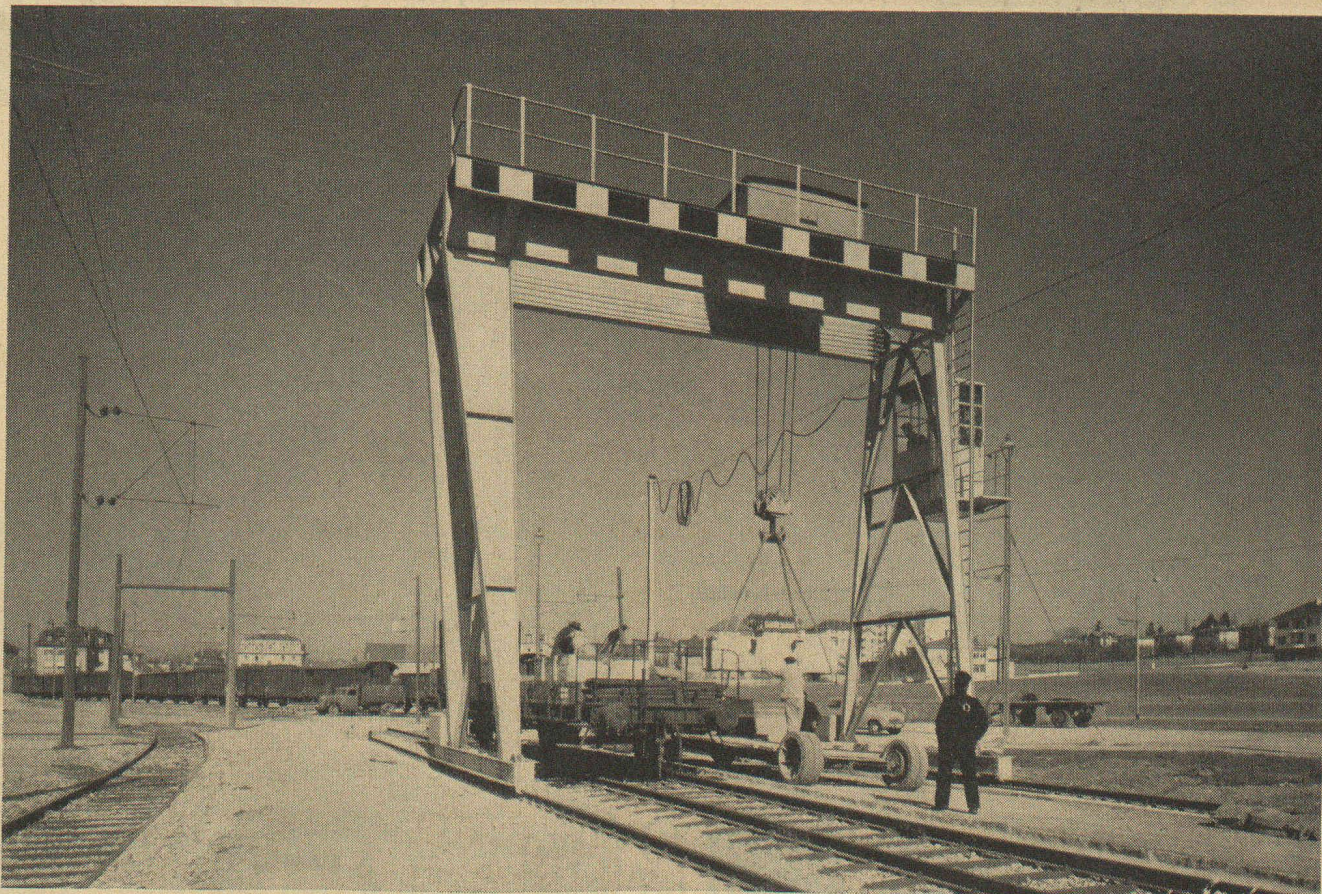
Grue à portique, capacité 25 T. — (Charpente métallique exécutée par ZWAHLEN & MAYR S. A.)
