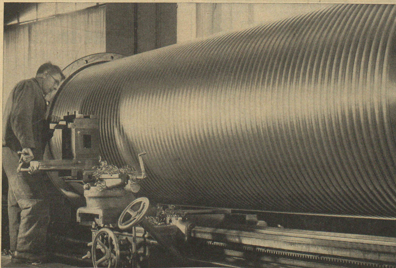
Tambour du treuil pour le funiculaire à matériel de l'Usine hydro-électrique souterraine des Clées (exécuté par les Ateliers de Constructions Mécaniques de Vevey S. A.)
