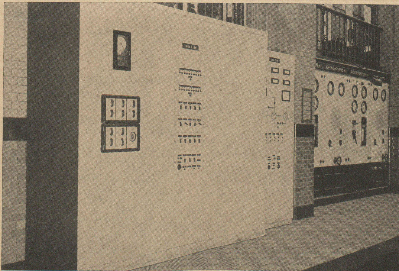
Installation de télécommande de réseau, livrée en Hollande (GEB Dordrecht), par LANDIS & GYR S. A., Zoug.
