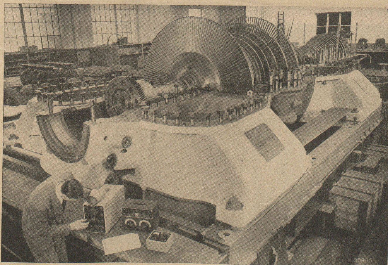
Mesure de vibrations sur une turbine à vapeur avec appareils PHILIPS
