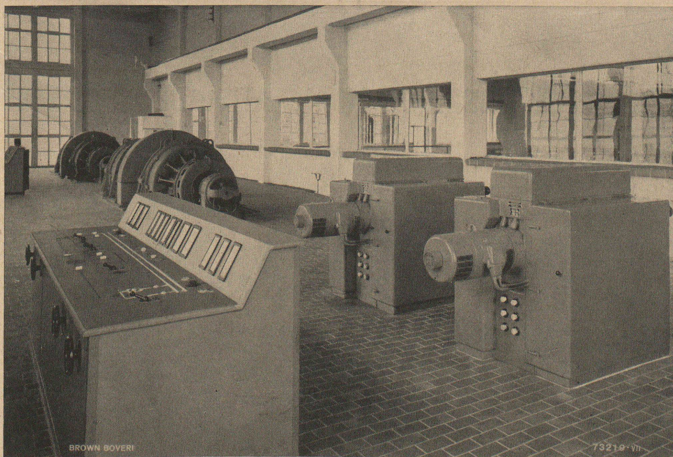
Convertisseurs à contacts Brown Boveri installés dans une usine chimique et pouvant débiter chacun 5000 A sous 150 à 230 V On voit au fond deux groupes convertisseurs rotatifs de 1500 kW chacun
