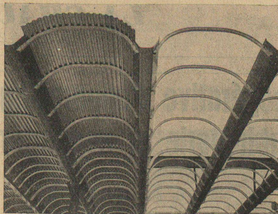
Avant-toit d'une entrée de gare. Voûtes en tonneau en bandes ondulées d'Aluman, profilées en arc et chéneaux autoportants en Anticorodal.
