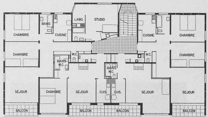
Fig. 63. — Etage 1 : 300.
