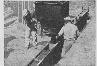
On coule le béton dans les éléments de coffrage.
