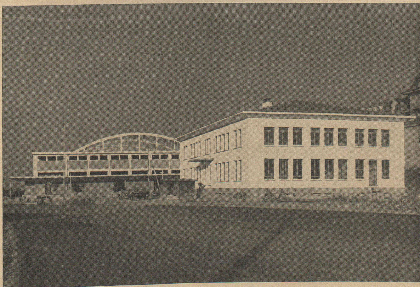
Les bâtiments de la nouvelle gare aux marchandises de Lausanne-Sébeillon. Au premier plan, le bâtiment de service, à peu près terminé. — A l'arrière plan, la halle aux marchandises. Les menuiseries extérieures de ces bâtiments ont été livrées par la FABRIQUE COOPÉRATIVE DE MENUISERIE DE LAUSANNE
