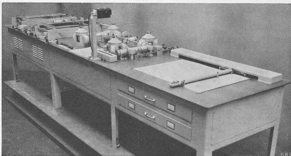
Fig. 14. Installation d'intégration pour le calcul automatique des trajectoires de projectiles. A l'avant, la table pour le tracé à l'échelle de la trajectoire.
