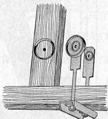
Demi-anneaux Assemblage de charpente en bois et fer
