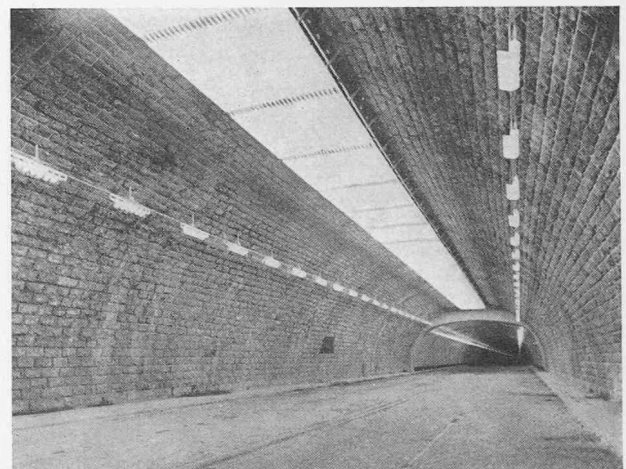
Fig. 17. — Entrée du tunnel routier de la Croix-Rousse, à Lyon. Sur les côtés, appareils à lampes 40 watts basse tension. Au plafond, 26 lignes de tubes haute tension.
