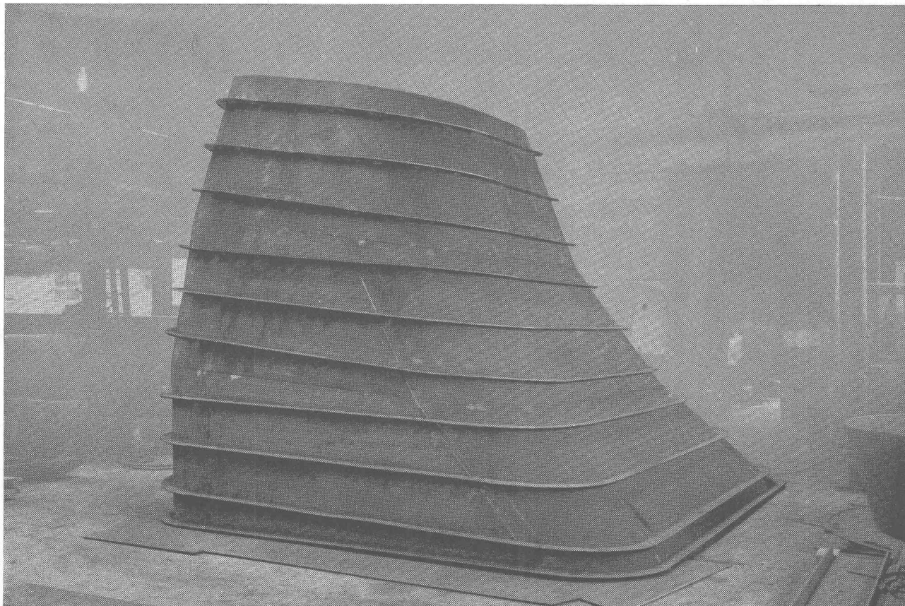
Usines des Clées. Blindage de la trompe d'entrée de la prise d'eau. — Exécution : Zwahlen & Mayr S. A., Lausanne.
