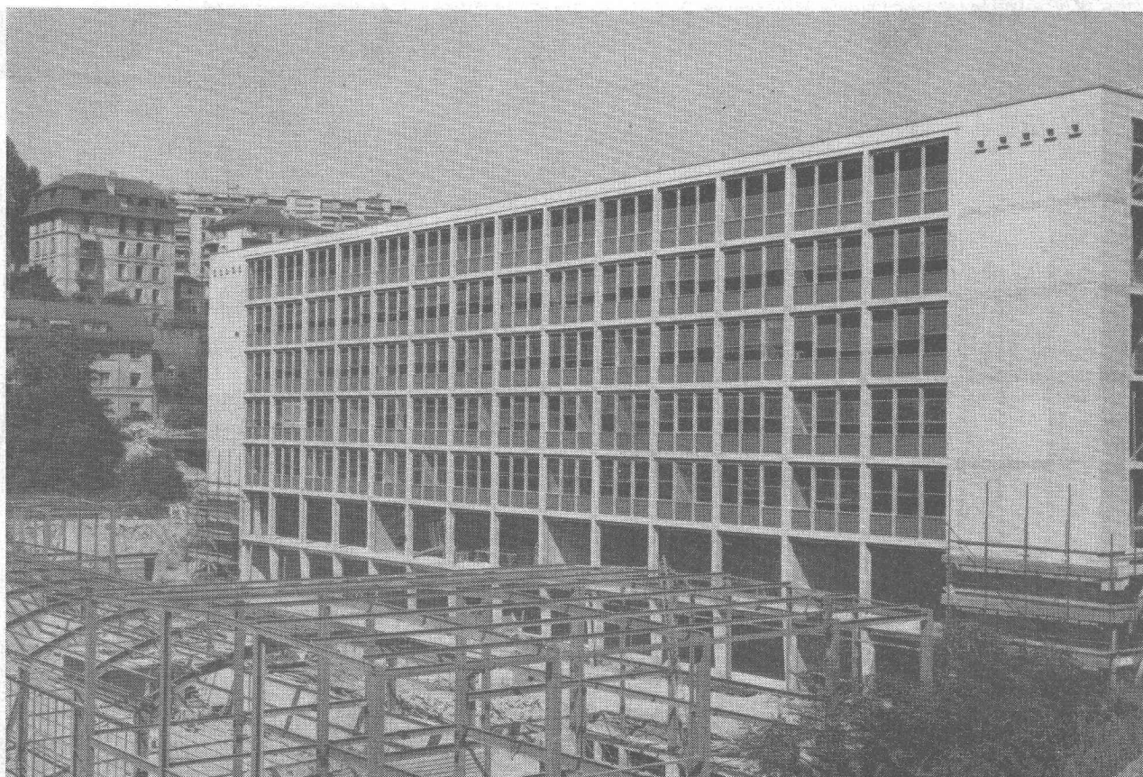
Bâtiment de l'Ecole Complémentaire Professionnelle à Lausanne. Fenêtres à double guillotine sans contrepoids (constructeur : ZWAHLEN & MAYR S. A.)
