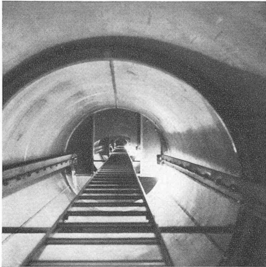
Fig. 8. — Eclairage de l'intérieur de la tour, avec plates-formes intermédiaires et montées des câbles électriques à gauche et à droite de l'échelle.
