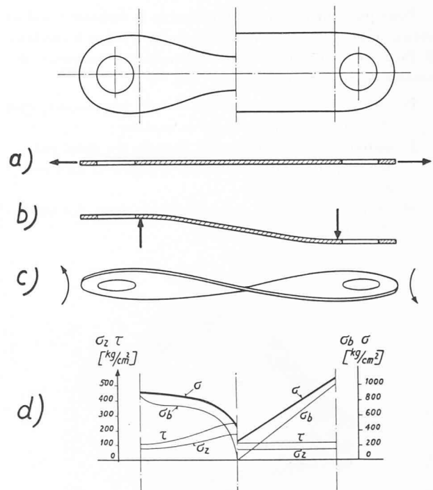
Fig. 3. — Sollicitation des lames de l'accouplement Sècheron. a = Traction. — b = Flexion. — c = Torsion. — d = Contraintes comparées des lames rectiligne et incurvée. \sigma_2 = contrainte de traction. — \sigma_b = contrainte de flexion. — \tau = contrainte de torsion. \sigma = contrainte combinée.
