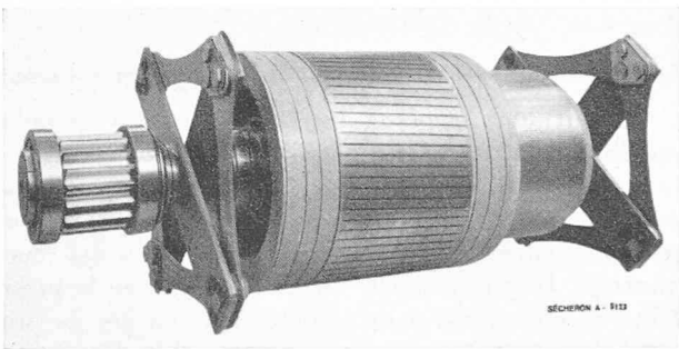
Fig. 2. — Transmission Sècheron à arbre à cardans, accouplements à lames et joints à créneaux.
