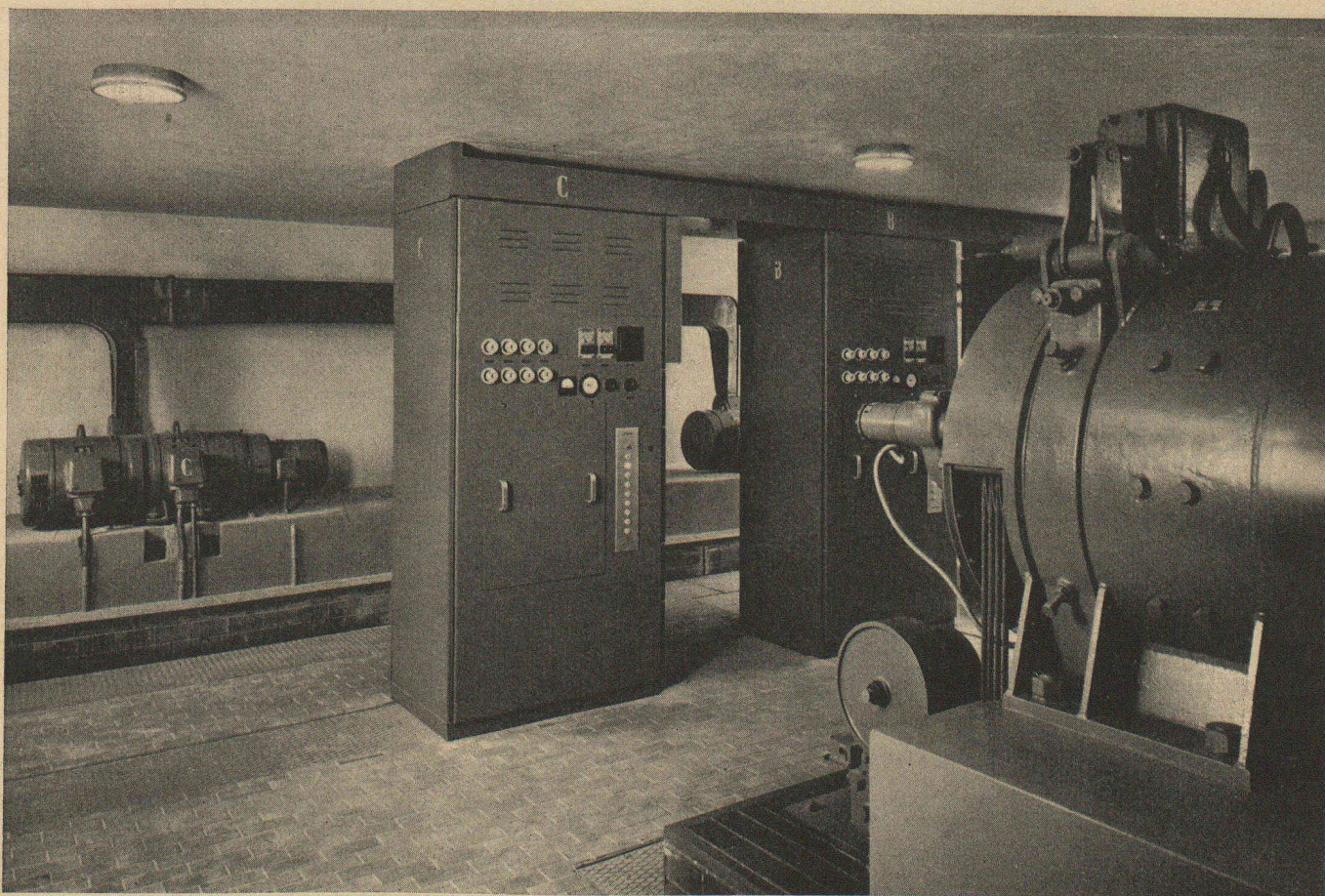
Salle de machines avec les armoires « VARIOTRON » d'une installation d'ascenseurs SCHLIEREN
