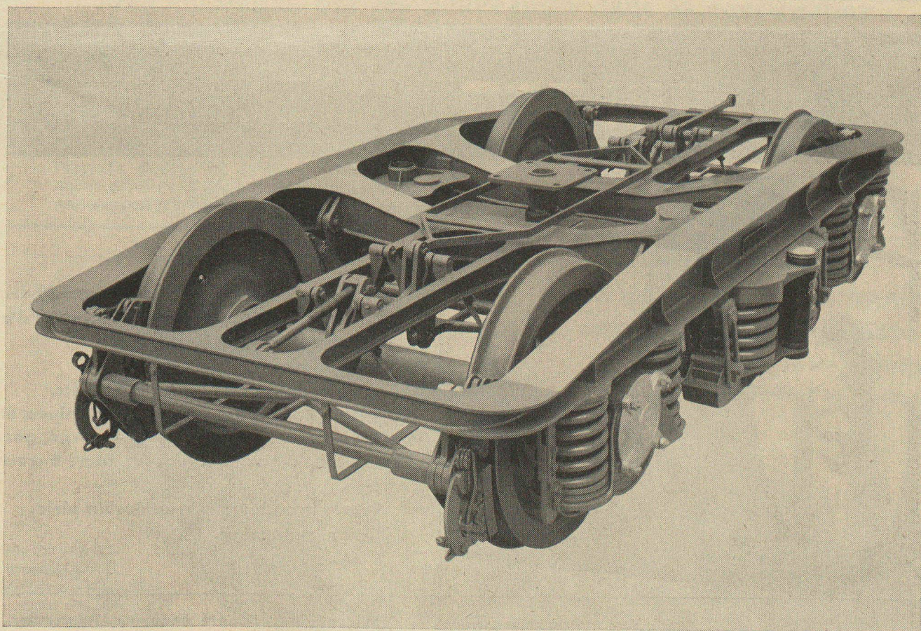
Bogie pour les wagons-lits de la Compagnie Internationale des wagons-lits construit par la Fabrique suisse de wagons et d'ascenseurs S. A., Schlieren-Zurich
