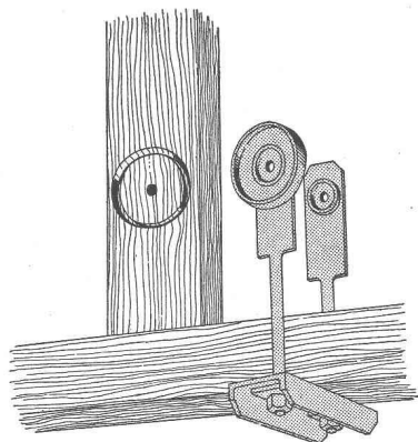
Demi-anneaux Assemblage de charpente en bols et fer
