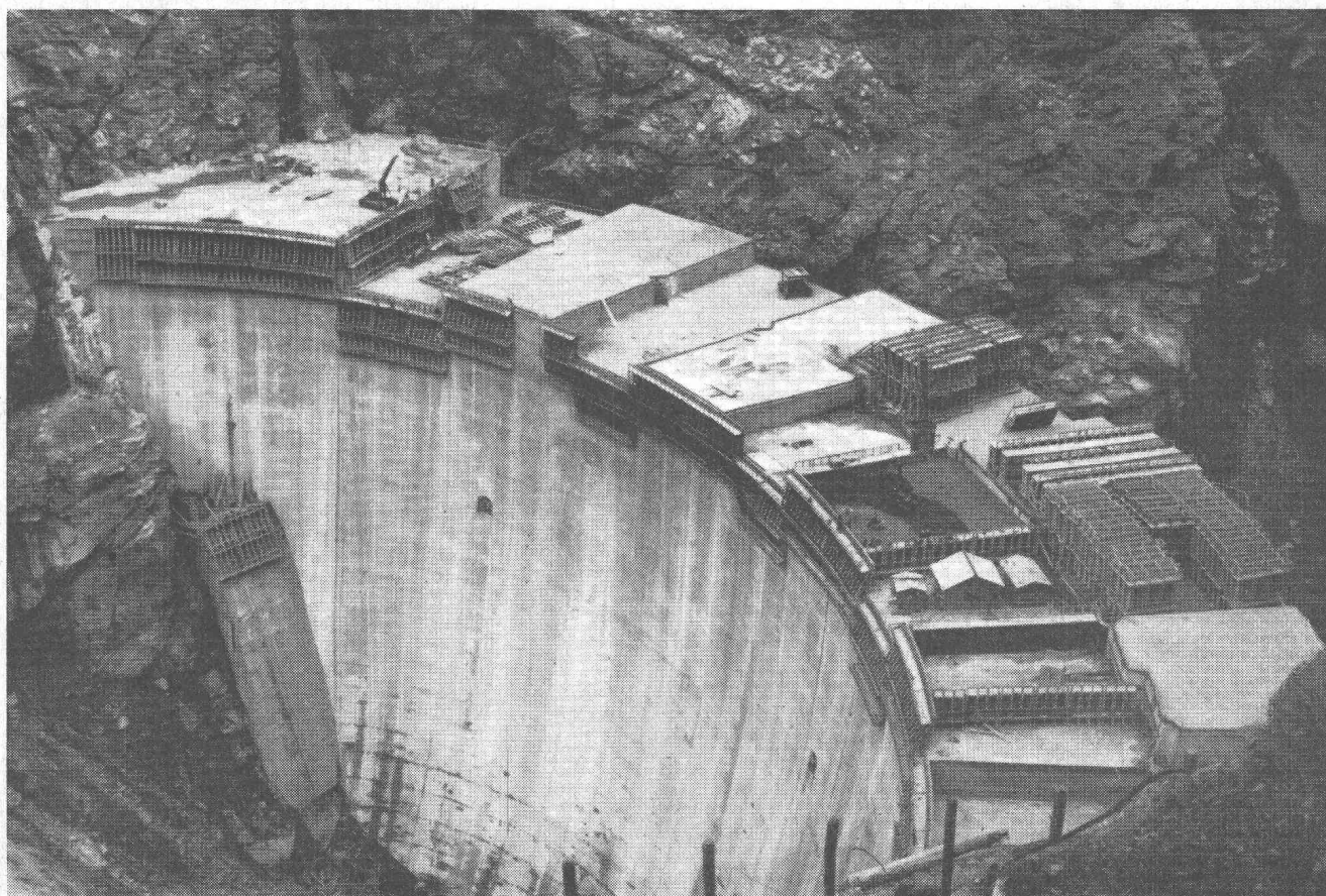
Barrage de Mauvoisin avec BARRA 55 - VINSOL. — Volume 2'000'000 m 3
