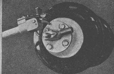
Contact ouvert, sans la calotte de protection.
