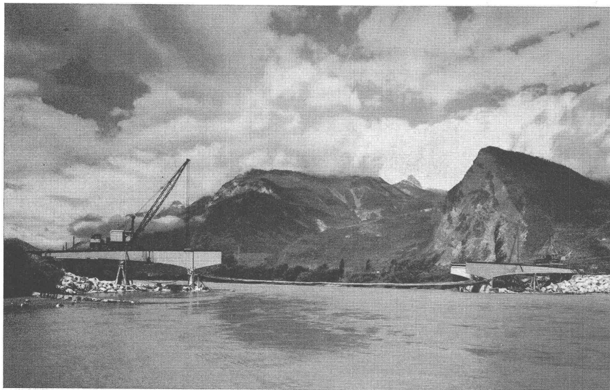
Pont-route en construction sur le Rhône, à Riddes.
