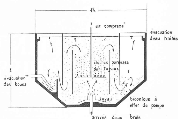
Fig. 5. — Le bloc d'épuration S.G.E.A.
