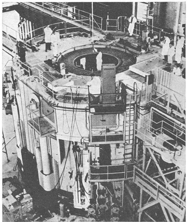
Fig. 3. — Réacteur NRX pendant la reconstruction. « Atomic Energy of Canada, Ltd. »
