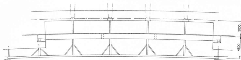
Fig. 6. — Plan d'ensemble du pont 3 de Mauvoisin.
