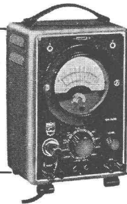
Millivoltmètre haute fréquence GM 6016
