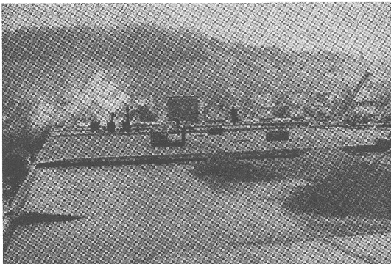
Etanchéité des toitures-terrasses des Usines PAILLARD à Ste-Croix, exécutée en asphalte souple multicouche par HIRSCHY & Cie S. A., Genève.
