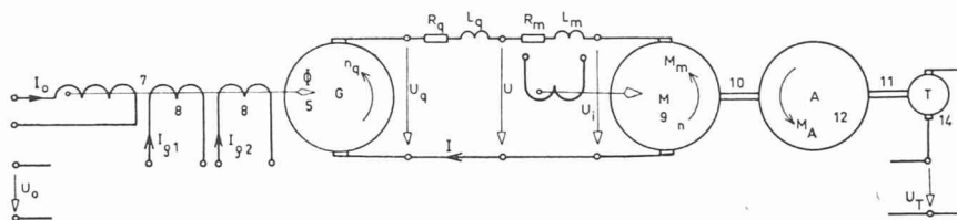
Fig. 22 a. — Groupe Ward-Leonard.
