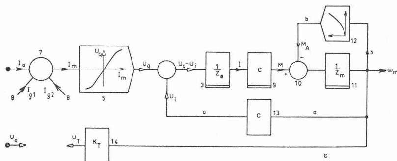
Fig. 22 b. — Schéma fonctionnel du groupe Ward-Leonard.
