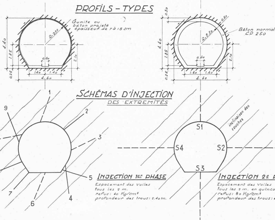
Fig. 3. Profils en travers type de la galerie et schémas d'injection
