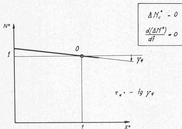
Fig. 9. — Courbe de statisme du régulateur de vitesse.
