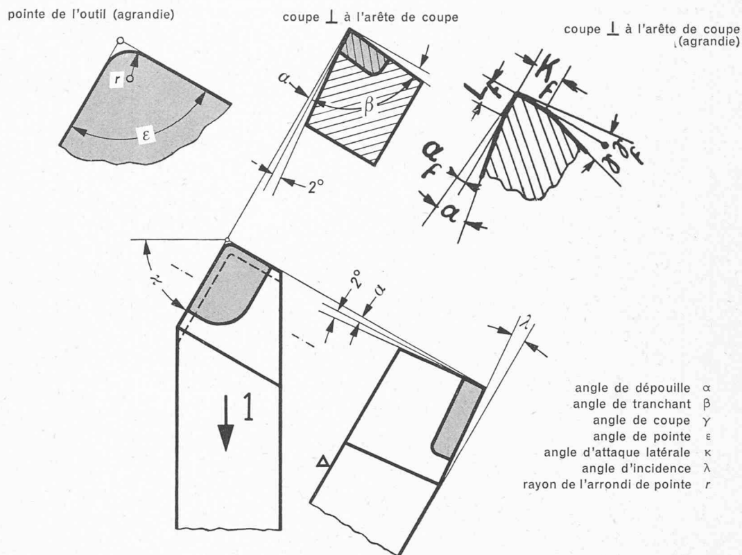
Fig. 5. — Angles de travail d'un burin.
