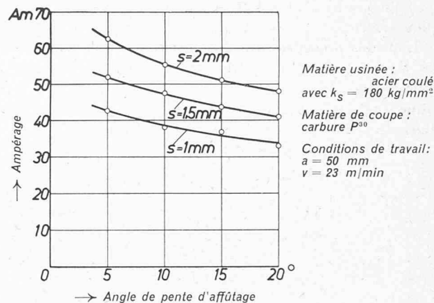
Fig. 6. — Ampérage d'un moteur de tour, en fonction de l'angle de coupe pour différentes avances.
