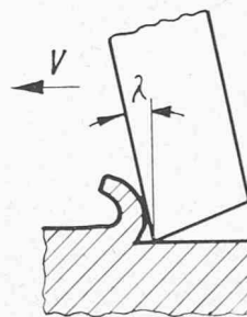
Fig. 7. — Couteau d'une fraiseuse avec coupe principale « suspendue » (négative).
