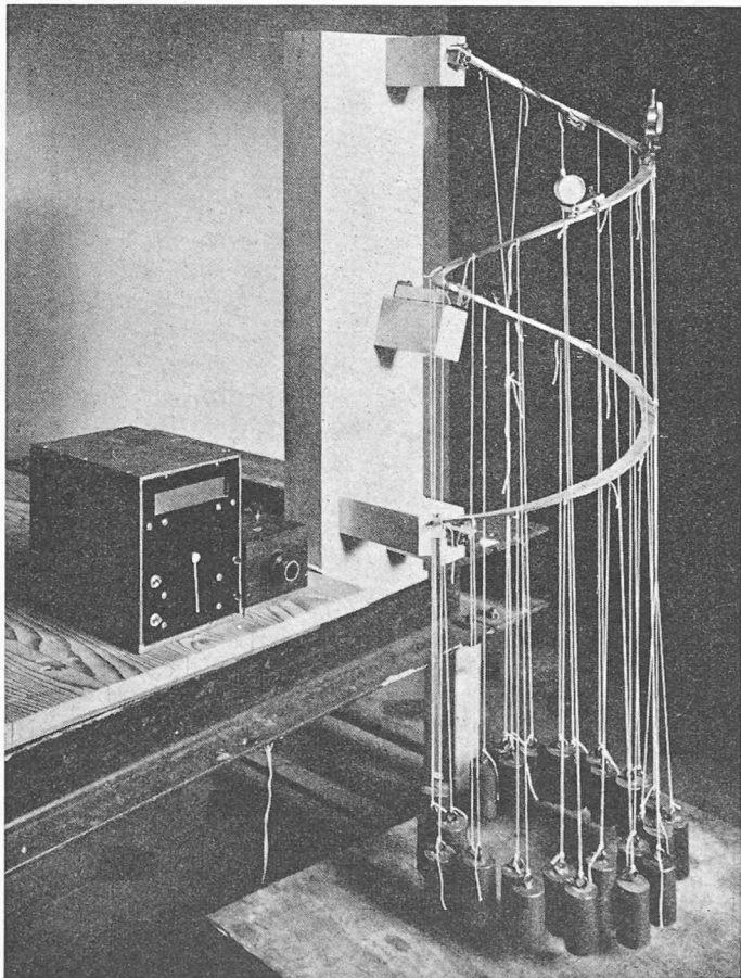
Fig. 2 b. — Modèle réduit. Barre de 5 × 20 mm en anticorodal.
