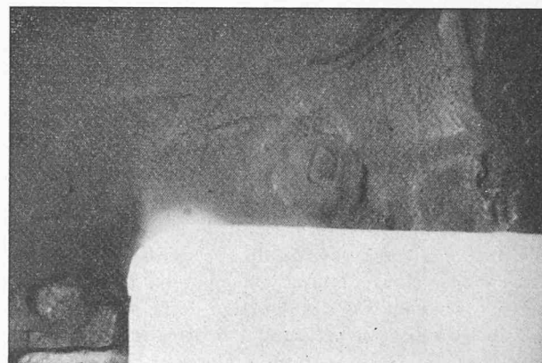
Fig. 12. — Formation d'un renard dans le limon bouillant micacé observé dans le chenal provisoire de drainage à l'amont du bassin.
