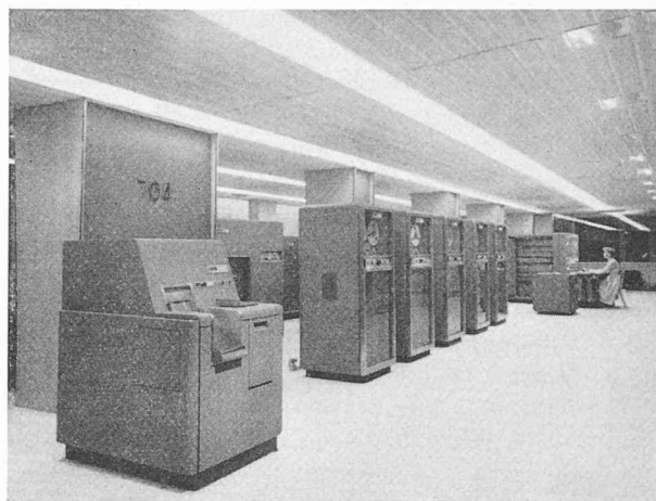
Fig. 2. — L'ordinateur IBM 704. Il comporte une mémoire centrale à tores magnétiques, des mémoires auxiliaires à tambours magnétiques et à bandes magnétiques.
